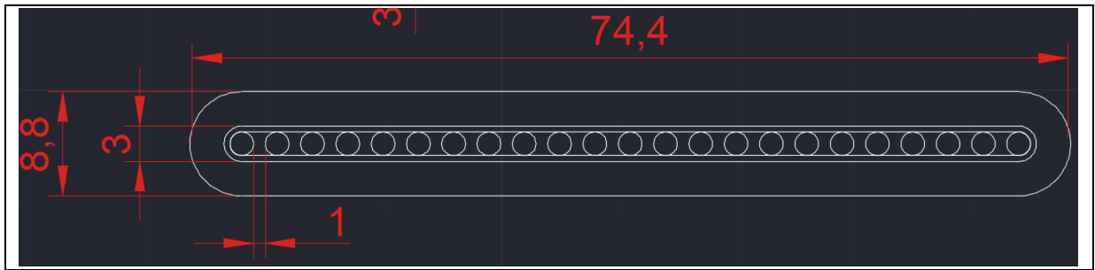
Figura 24 – Schema scavo
