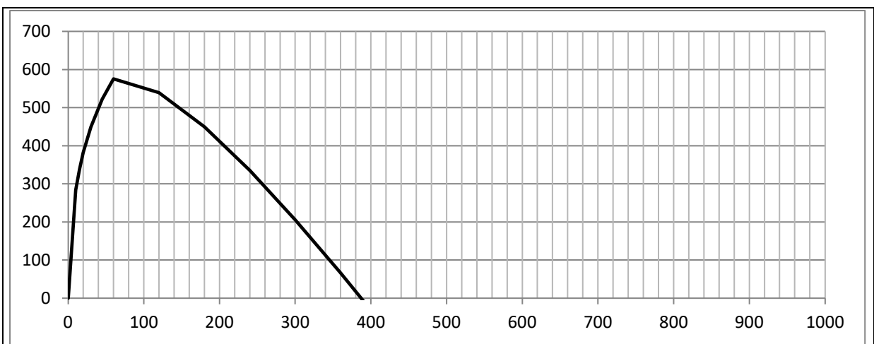
Figura 25 - Andamento afflussi-deflussi con Tr=100 anni
