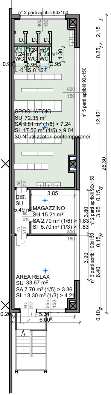
V4 Piano Primo 1:200
