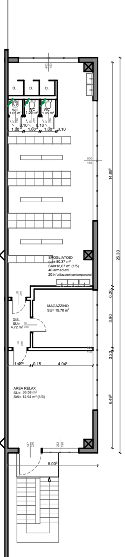
AUTORIZZATO V2 PIANO PRIMO 1:250
