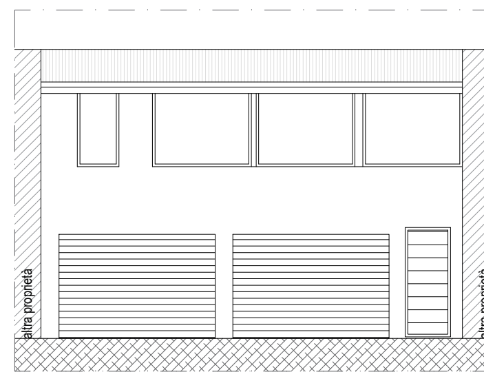
Sezione A-A
