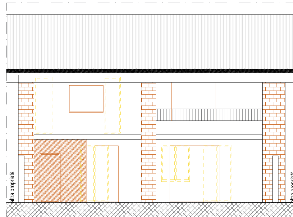
Prospetto SUD
