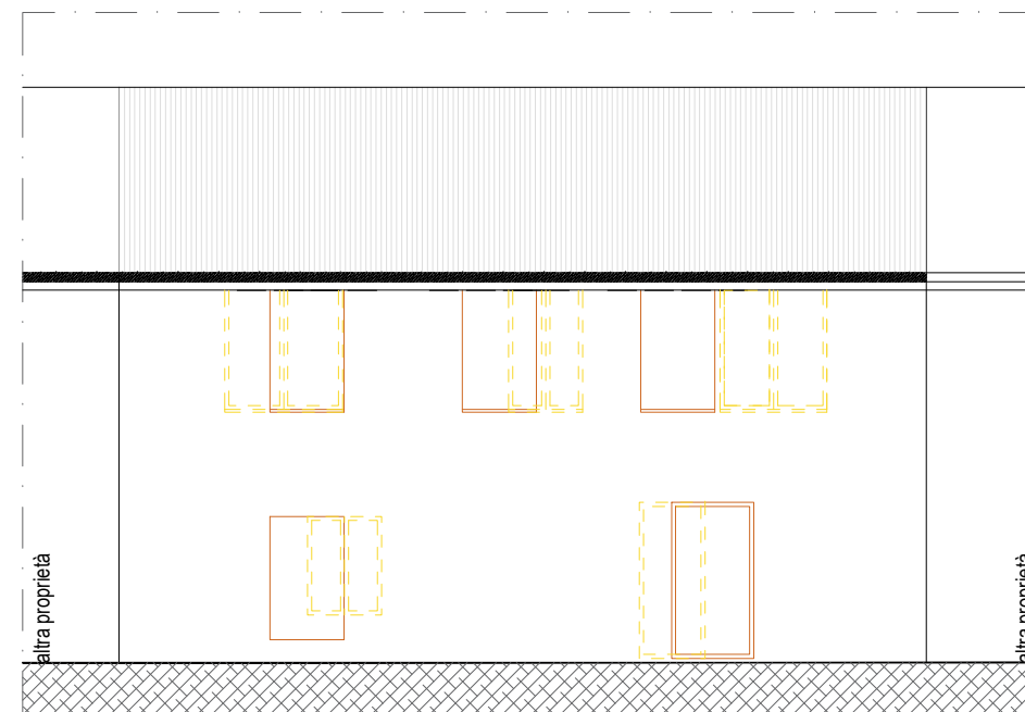
Sezione A-A
