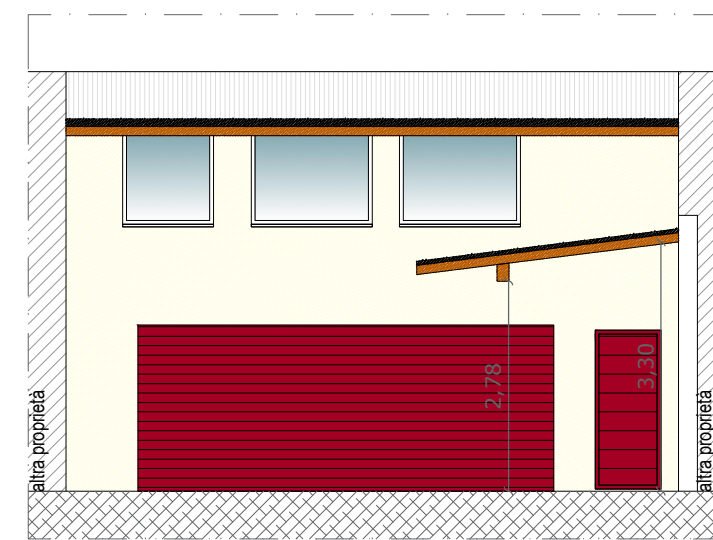
Sezione A-A
